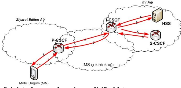
Şekil 4: 8 mesajdan oluşan IMS eldeğiştirme şeması
