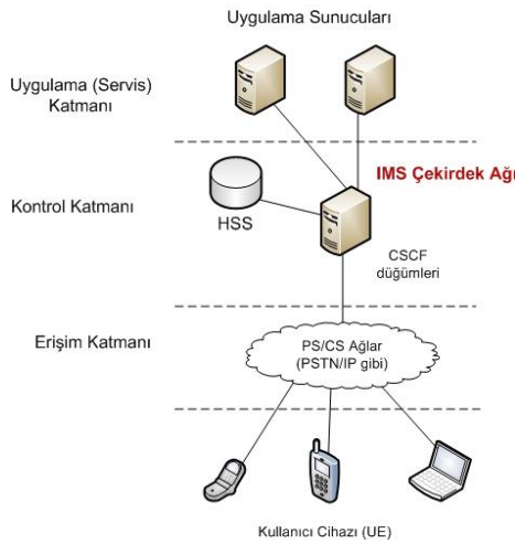
Şekil 1: IMS Katmanlı Yapısı
