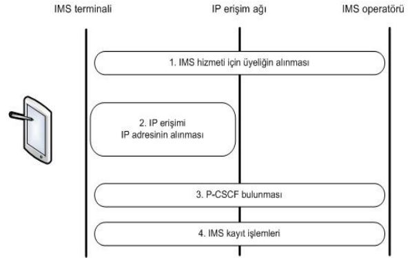
Şekil 2 Hizmet almak için gerekli adımlar IMS kayıt işlemleri SIP REGISTER mesajı ile gerçekleştirilir.
