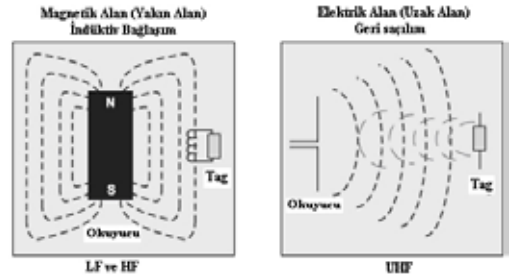
Şekil 4. RFID Anten türleri
