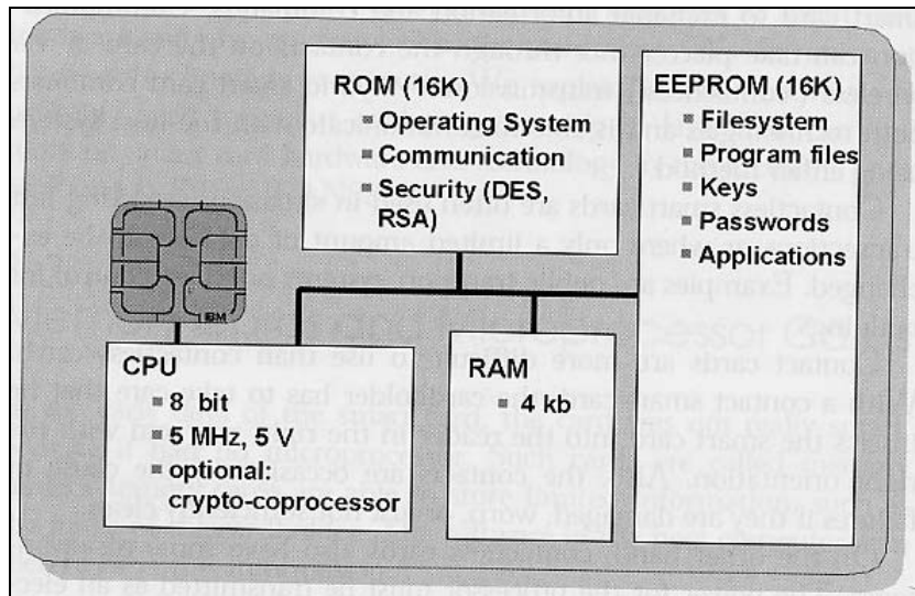
Şekil 2.1: Bir akıllı kart entegresi ve bileşenleri (Hansmann et al., 2000)
