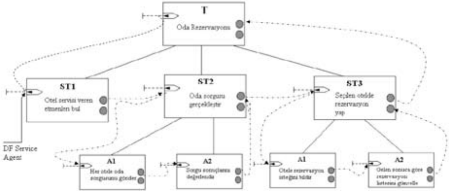
Şekil 4. Oda Rezervasyonu görevine ait HTN yapısı
