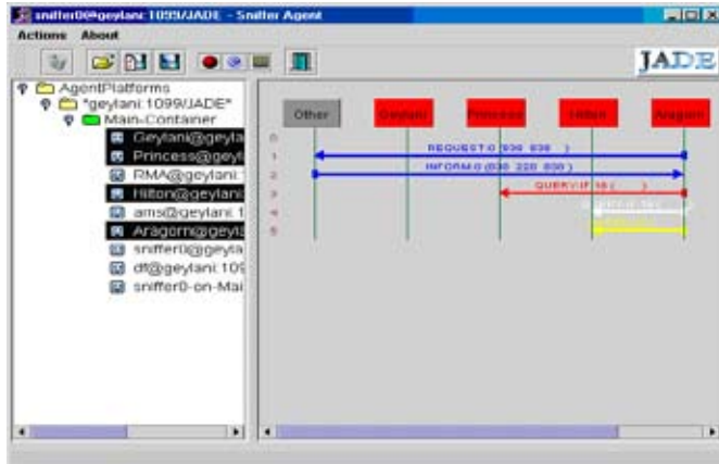
Şekil 5. JADE Sniffer (Yoklayıcı) etmeni kullanarak etmen iletişimlerinin gözlenmesi
