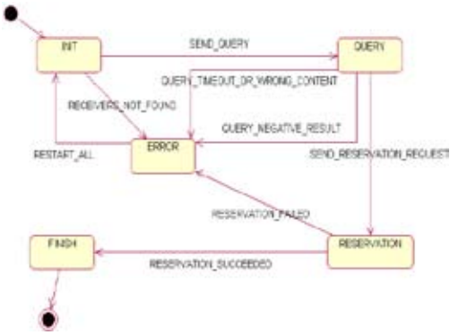
Şekil 2. CustomerAgent etmeninin FSM yapısındaki davranış modeli
