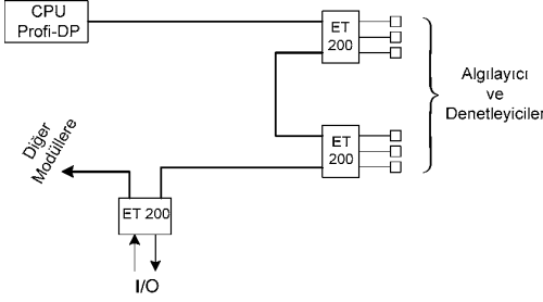
Şekil 1. Profibus-DP ağ yapısı
