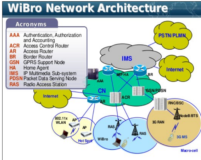
Şekil 5 - WiBro Ağ Mimarisi [3]
