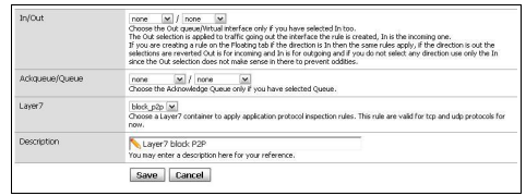
Resim 2. Firewall kural yazım alanı
