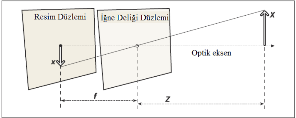
Şekil 3. İğne delikli kamera modeli
