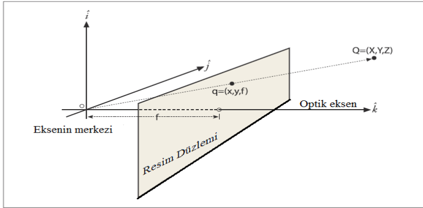
Şekil 4. Resim Düzlemi, eksen merkezi ilişkisi
