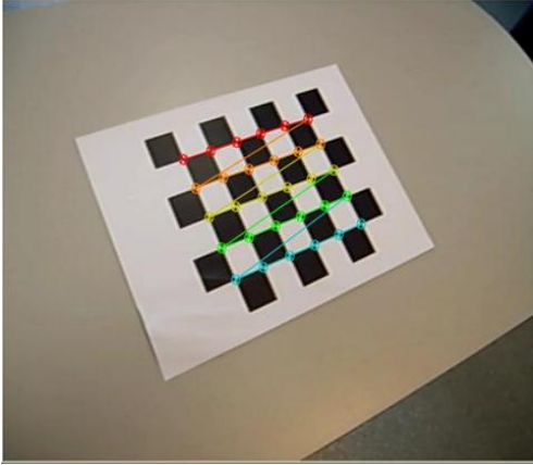
Şekil 7. Satranç tahtası resmine cvDrawChessboardCorners() fonksiyonunun uygulanışı
