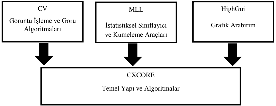
Şekil 1. OpenCV Bileşenleri
