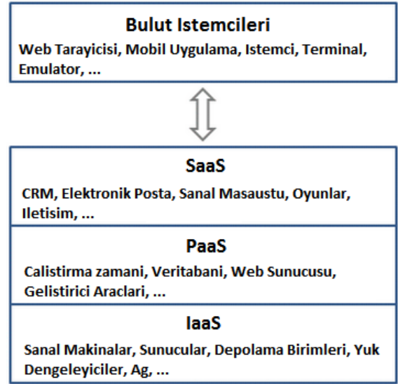
Sekil 2 - Bulut Bilişimin Servis Modelleri [2]
