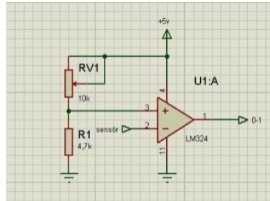
Şekil 7. IR Sensörlü gerilim bölücü devresi.
