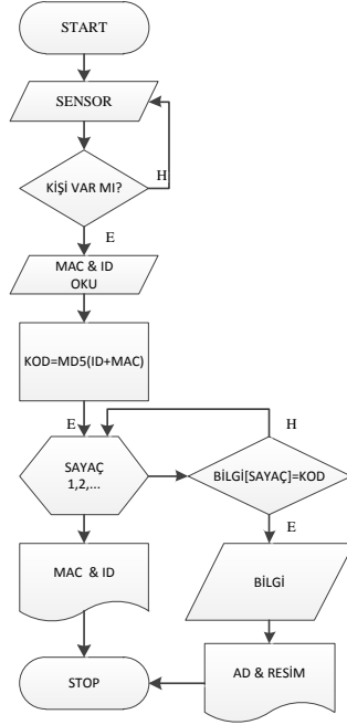
Şekil.6 Akış diyagramı.
