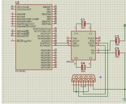
Şekil.8 Mikrodenetleyici seri iletişim şeması.
