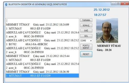
Şekil.7 PC arayüzü.
