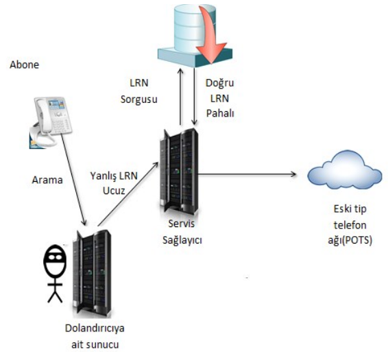
Şekil 8: Konum Yönlendirme Numarası Dolandırıcılığı [2]
