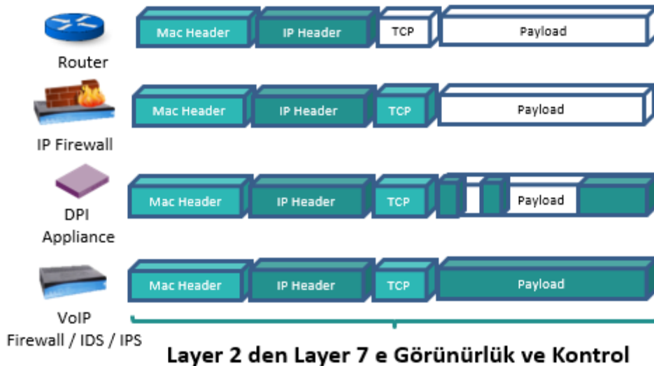
Şekil 3. Güvenlik Ürünleri ve Paket Analiz Düzeyleri
